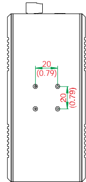
后视图
