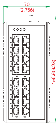
前视图
